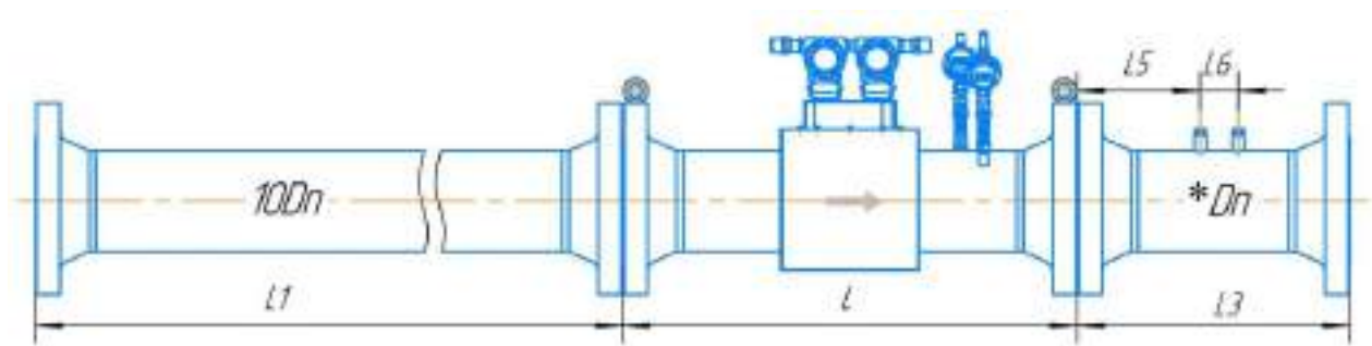
Рисунок Д.36 – Монтаж расходомера класса точности В/В*±1,0/1,2* (1,5)* для исполнения с дублированием по стандарту ASME B16.5-2003
