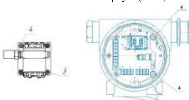
Рисунок 24 – Выносной терминал в металлическом корпусе (ВТМ)
