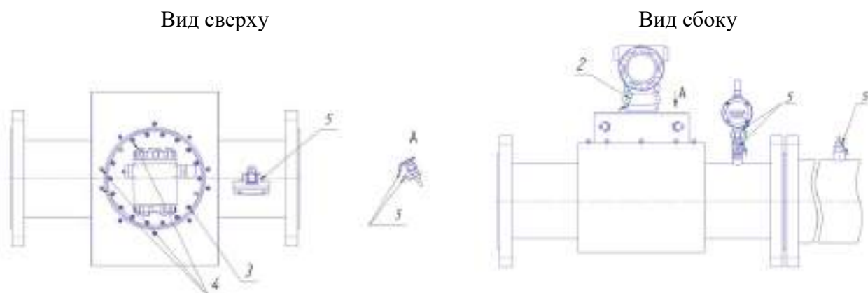
Рисунок 20 – Корпус круглого сечения с защитным кожухом
