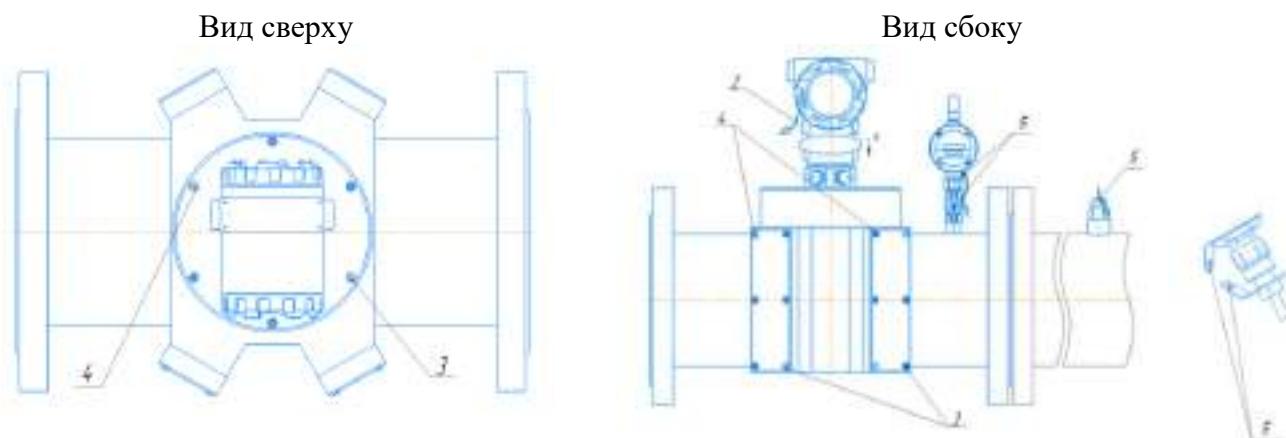
Рисунок 18 – Корпус круглого сечения с отдельными защитными крышками
