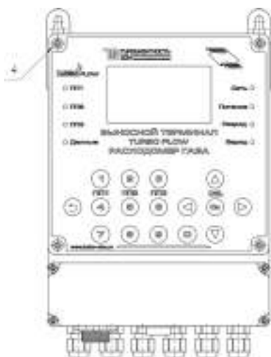
Рисунок 23 – Выносной терминал (ВТ)
