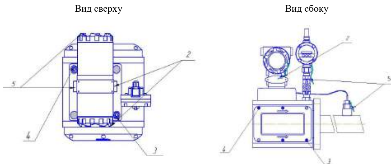
Рисунок 19 – Корпус прямоугольного сечения с совмещенными защитными крышками
