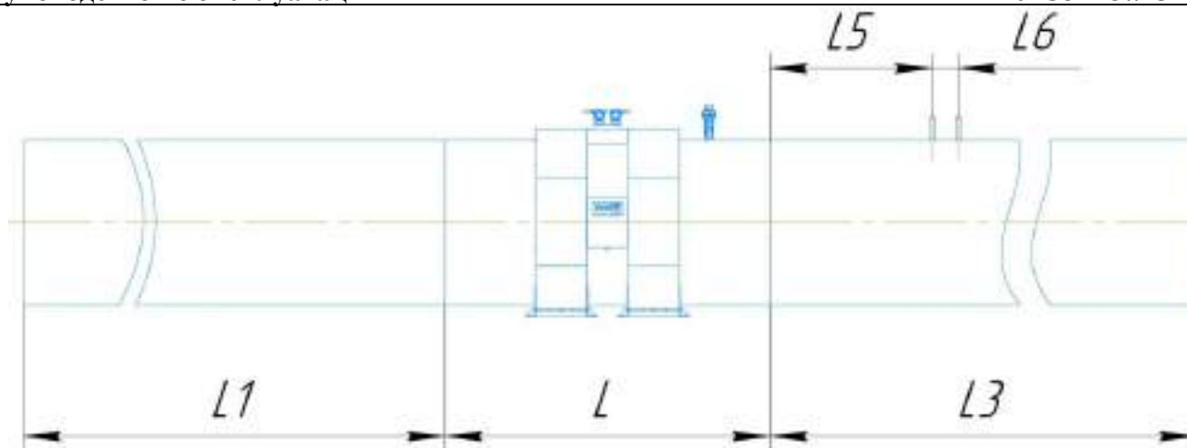
Рисунок Д.40 – Монтаж расходомера классов точности A/A^* \pm 0,5/0,7^*(0,7)^* и B/B^* \pm 0,5/0,7^*(0,7)^* для бесфланцевого исполнения с дублированием
