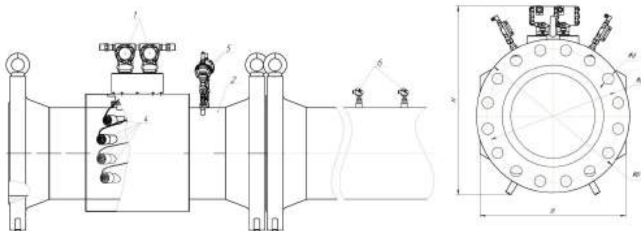
Рисунок Б.11 - Расходомер - счетчик газа ультразвуковой исполнение с дублированием дБ
