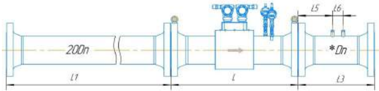
Рисунок Д.32 – Монтаж расходомера классов точности A/A^* \pm 0,5/0,7^*(0,7)^* и B/B \pm 0,5/0,7^*(0,7)^* для исполнения с дублированием по стандарту ASME B16.5-2003
