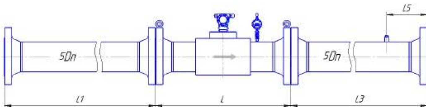
Рисунок Д.23 – Монтаж реверсивного расходомера класса точности G/I^* \pm 2,0/2,2^* (2,5)^* или \pm 1,0/1,2^* (1,5)^* для исполнения корпуса VR по стандарту ASME B16.5-2003
