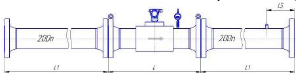
Рисунок Д.21 – Монтаж реверсивного расходомера классов точности А/А*±0,5/0,7*(0,7)* и Б/Б ±0,5/0,7*(0,7)* для исполнения корпуса VR по стандарту ASME B16.5-2003
