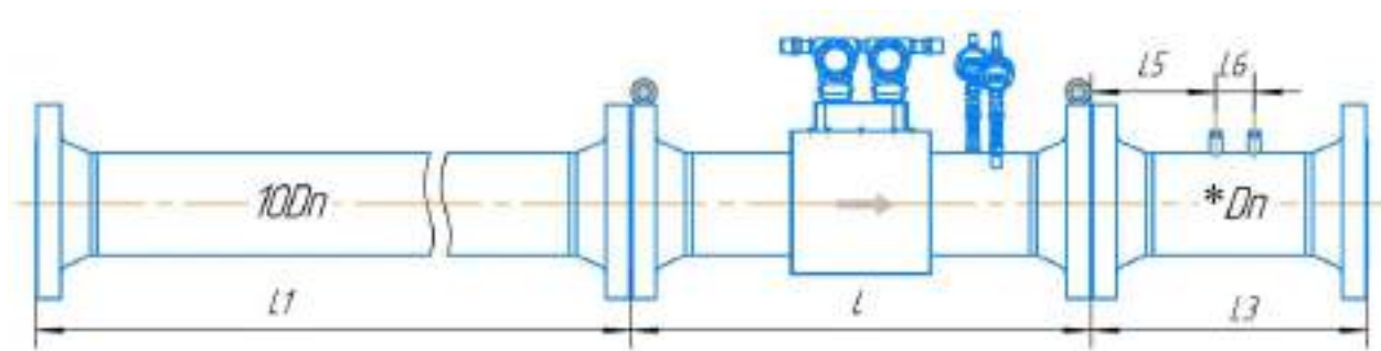
Рисунок Д.36 – Монтаж расходомера класса точности V/B^* \pm 1,0/1,2^* (1,5)^* для исполнения с дублированием по стандарту ASME B16.5-2003
