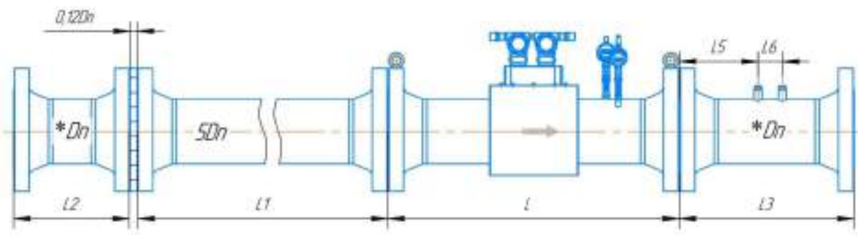
Рисунок Д.34 – Монтаж расходомера со струевыпрямителем укороченной длины со вставкой 2 Dn классов точности А ±0,5 и Б ±0,5 для исполнения с дублированием по стандарту ASME B16.5-2003
