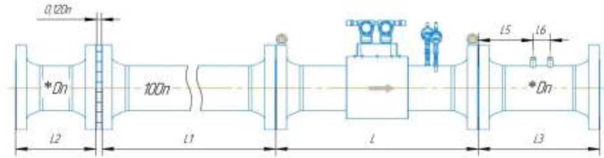
Рисунок Д.33 – Монтаж расходомера со струевыпрямителем со вставкой 2 Dn классов точности А/А*±0,5/0,7*(0,7)* и Б/Б ±0,5/0,7*(0,7)*
