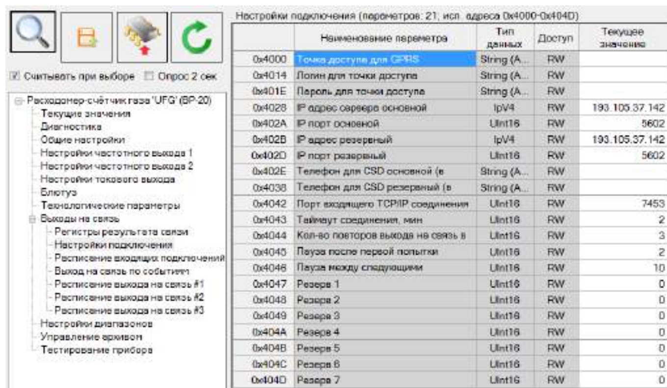
Рисунок 2.87 – Настройки подключения
