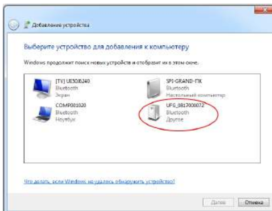
Рисунок 2.25– Добавление устройства
