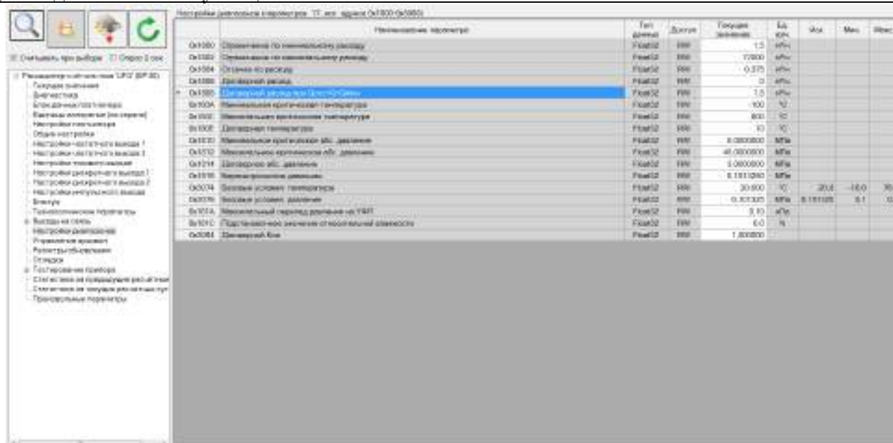
Рисунок 2.50 – ЭФ "Параметры"
