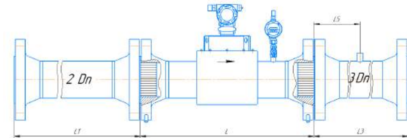
Рисунок Д.42 – Монтаж расходомера класса точности V/V^* \pm 1,0/1,2^* (1,5)^* с УФП С1 для исполнения корпуса V и С с типом присоединительных фланцев по ГОСТ 33259
