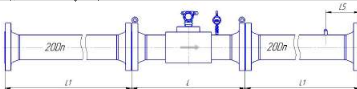
Рисунок Д.12 – Монтаж реверсивного расходомера классов точности A/A^* \pm 0,5/0,7^*(0,7)^* и B/B^* \pm 0,5/0,7^*(0,7)^* для исполнения корпуса VR и CR с типом присоединительных фланцев по ГОСТ 33259
