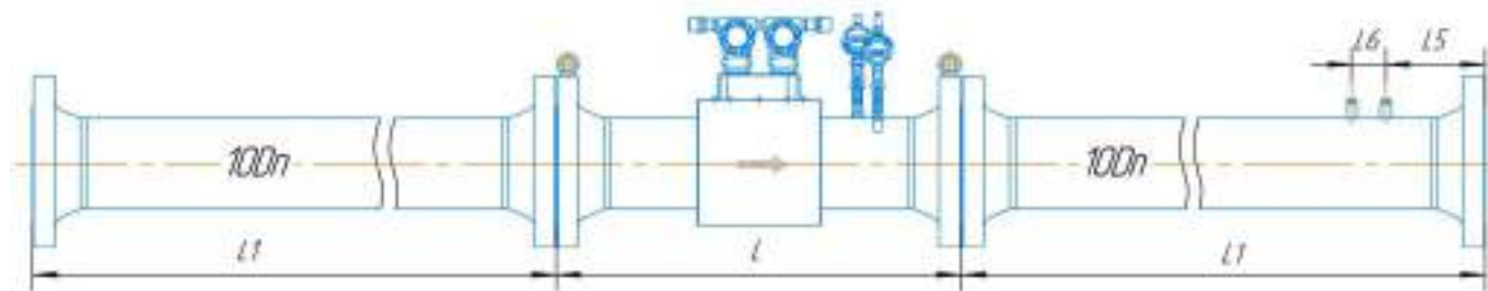
Рисунок Д.31 – Монтаж реверсивного расходомера класса точности B/B^* \pm 1,0/1,2^* (1,5)^*
